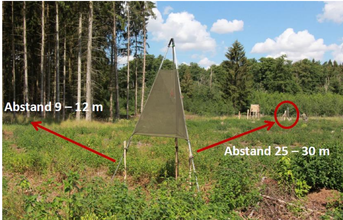
Abb. 1: Korrekte Platzierung von Trinet P Fangsystemen (Mindest- und Maximalabstände zu Fichten sowie zwischen den einzelnen Trinet P Fangsystemen)
