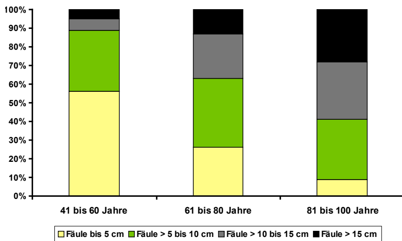
Abb. 5: Fäuledurchmesser am Stock (in Klassen) und Alter der Bäume in Form von Altersklassen.
