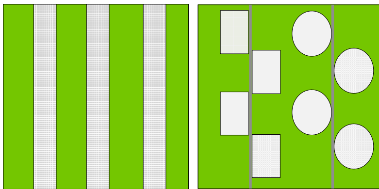
Abb. 10: Schematische Darstellung von Kulissen- (links) und Lochhieben (rechts) in Erlenbeständen: Helle Flächen werden genutzt, grüne verbleiben bis zur Etablierung des Folgebestandes als Rückzugsräume für typische Arten der Bruchwälder. Die etwa 50-60 m breiten Kulissen werden streifenförmig, die rund 0,3 - 0,5 ha großen Löcher als rechteckige bzw. kreisförmig-ovale Flächen entlang der Bringungslinien (dunkelgrau) angelegt.
