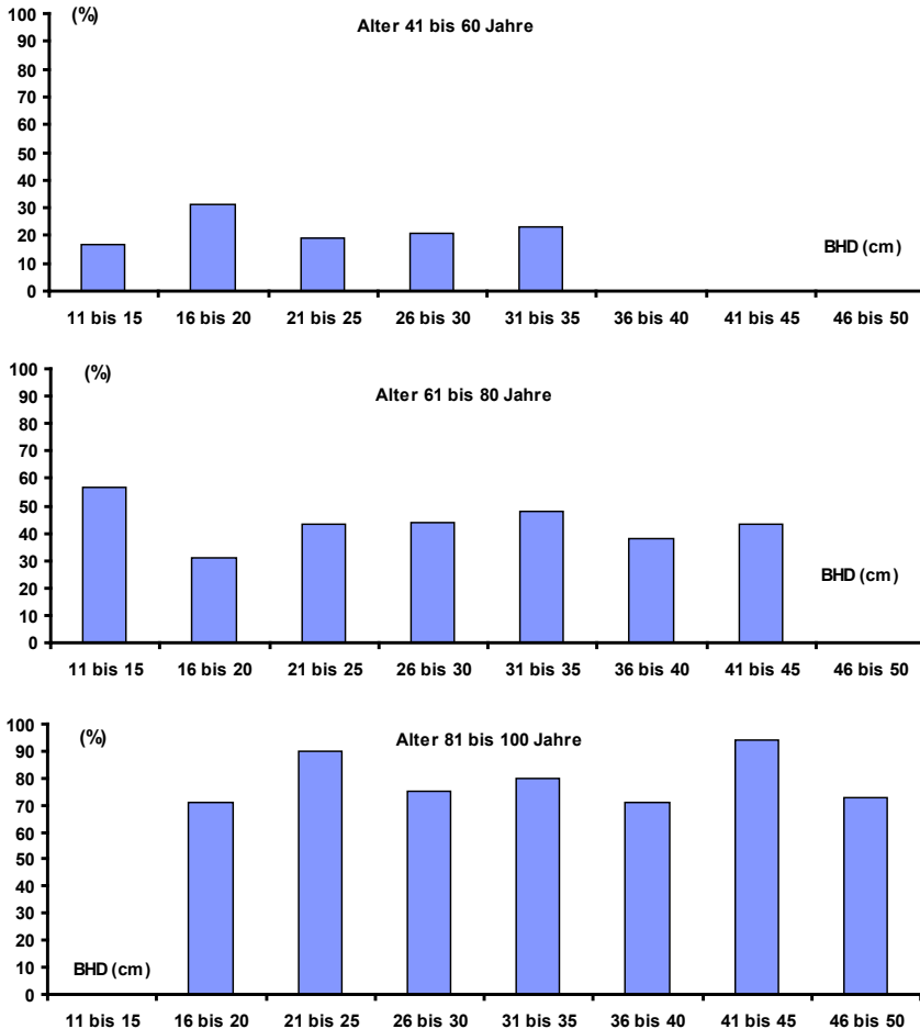
Abb. 4: Kernfäulebefall und Brusthöhendurchmesser für Bäume der Altersklasse III (Alter 41 bis 60 Jahre), Altersklasse IV (Alter 61 bis 80 Jahre) und Altersklasse V (Alter 81 bis 100 Jahre).
