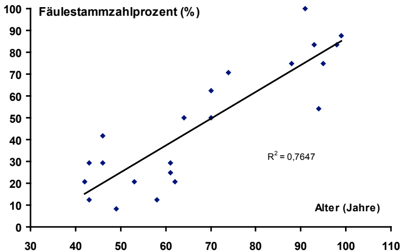
Abb. 3: Fäulestammzahlprozent in Abhängigkeit vom Alter der Bestände.
