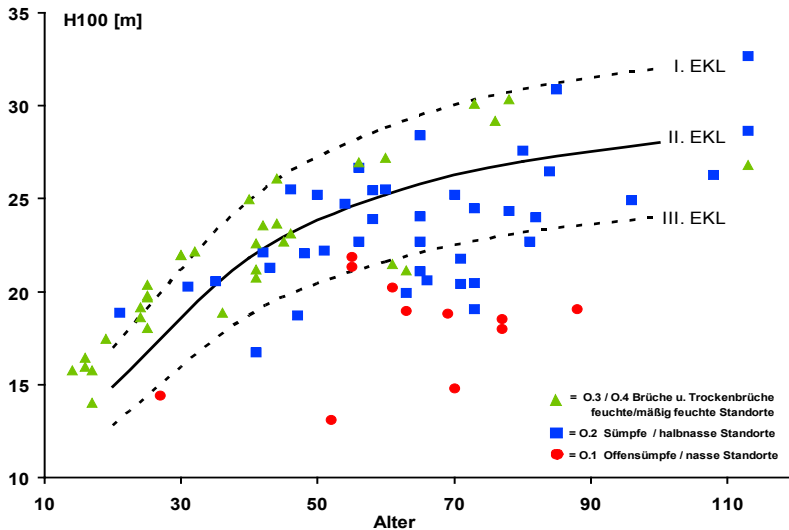
Abb. 6: Oberhöhe (H100) von Erlenprobebeständen auf Moorstandorten mit unterschiedlichem Grundwassereinfluss. Als Bezugsmaßstab sind die Ertragsklassen (EKL) I, II und III der Roterlen-Ertragstafel 1994 von LOCKOW eingezeichnet (aus SCHRÖDER 2005).
