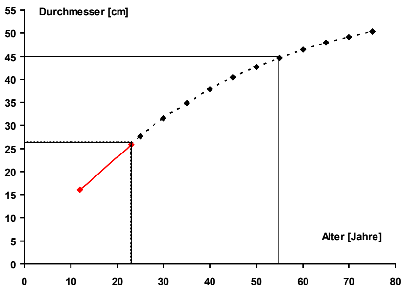
Abb. 8: Durchmesserentwicklung von Erlen-Z-Bäumen als „Ist“ (Durchschnittswerte der Z-Bäume des Weiserbestandes vom Alter 12 bis 23 Jahre) und als Prognose (Zuwächse des Oberdurchmessers der Ertragstafel ab Alter 24).
