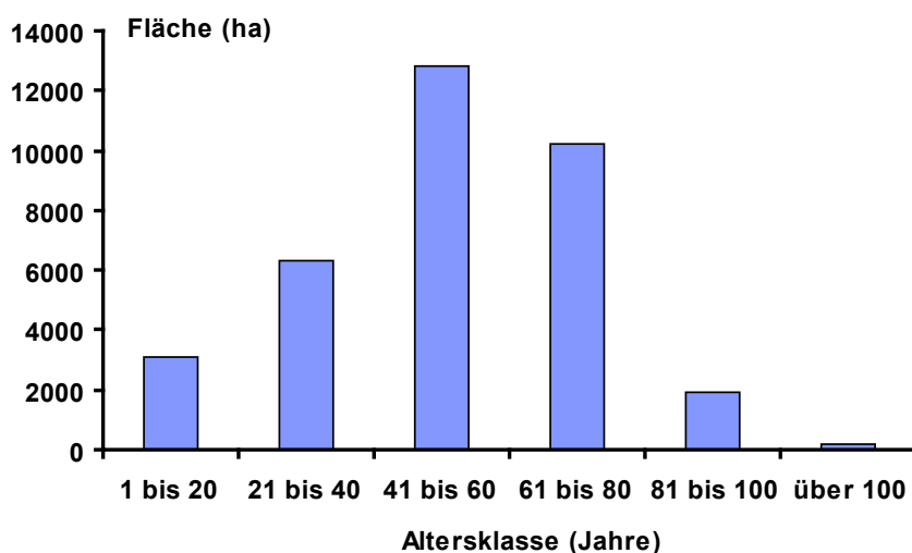
Abb. 1: Altersflächenverteilung der Roterle nach Altersklassen.
