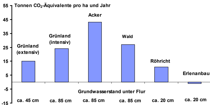
Abb. 9: Klimarelevanz von Mooren unter verschiedenen Nutzungsformen, wobei Röhricht und Erlenanbau den Zustand nach Wiedervernässung auf mind. 20 cm unter Flur beschreiben (nach MLUV M-V 2009, Konzept zum Schutz und zur Nutzung der Moore).
