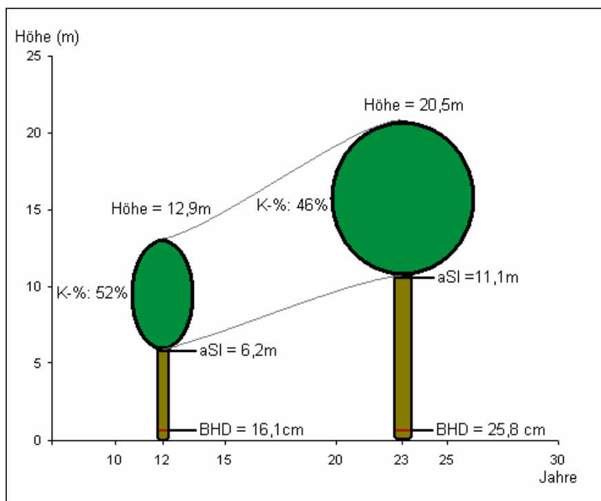
Abb. 7: Kennwerte von Z-Bäumen in Form von Durchschnittswerten eines Weiserbestandes im Alter von 12 Jahren (1. Aufnahme) und im Alter von 23 Jahren (2. Aufnahme).
